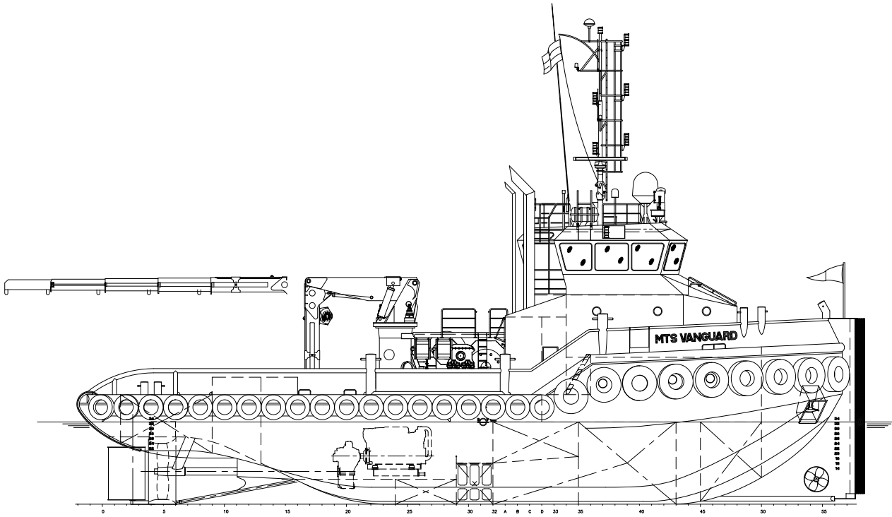
Maindeck
